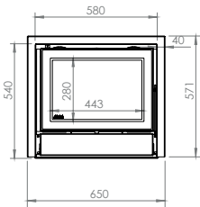
NORDIC PLUS 58/54
