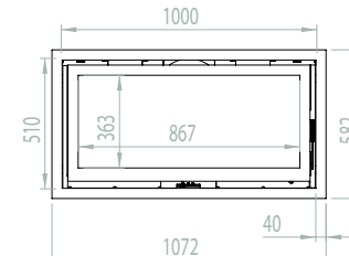
PURE 16/9
