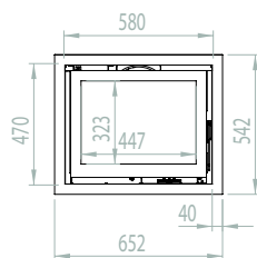
PURE 58/47
