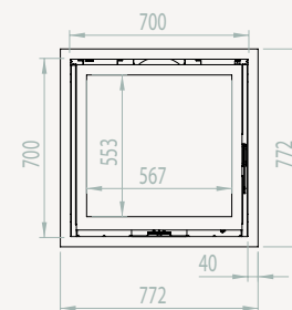
PURE 70/70
